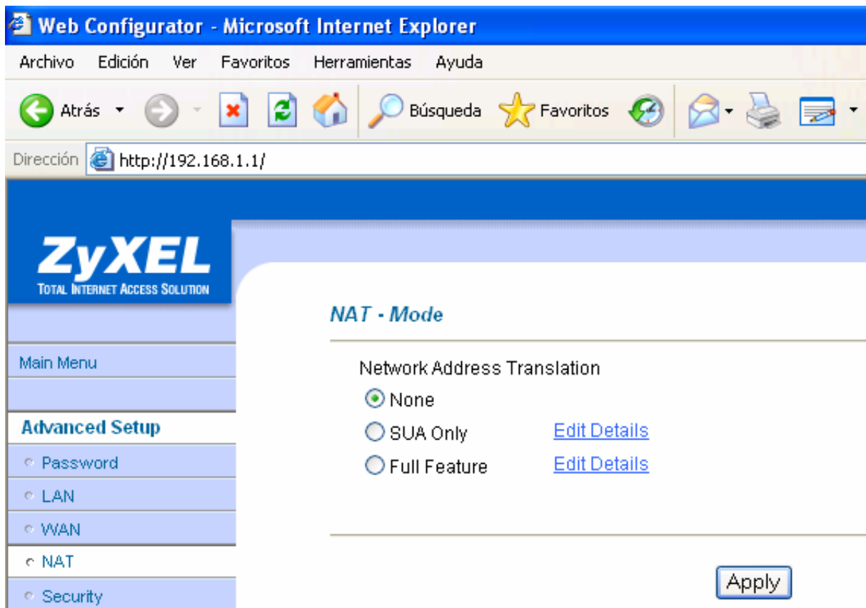
Figura 3-6: NAT deshabilitado
